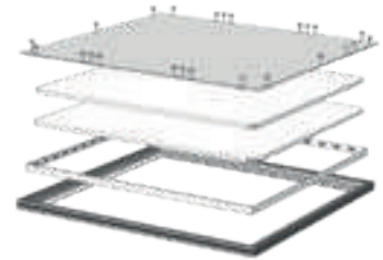
Opbouw LED-paneel
